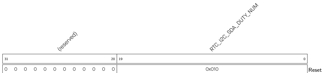
Register 2.16. RTC_I2C_SDA_DUTY_REG (0x0018)
