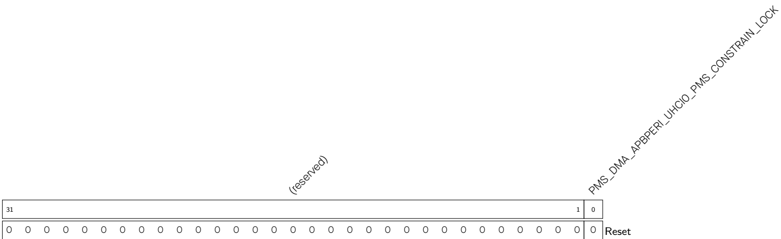
Register 15.10. PMS_DMA_APBPERI_UHCIO_PMS_CONSTRRAIN_O_REG (0x0048)
