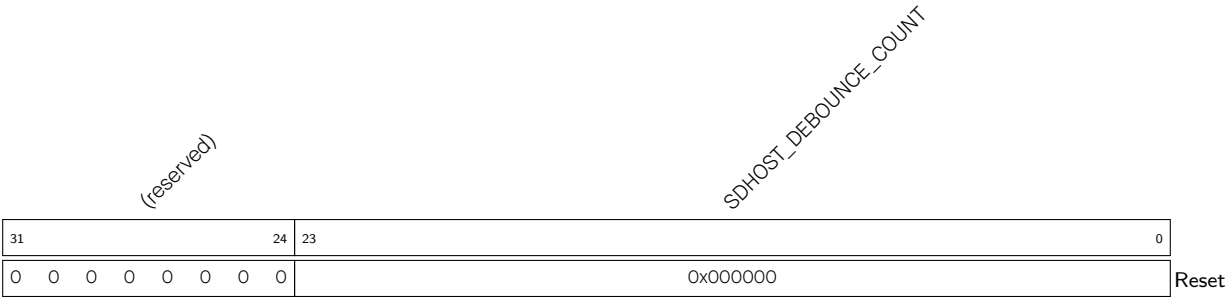
Register 34.24. SDHOST_DEBNCE_REG (0x0064)
